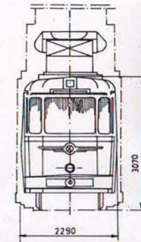
6.1. ábra. 1200-as pályaszámú csuklós motorkocsik jellegrajza és fontosabb berendezéseinek elhelyezése
