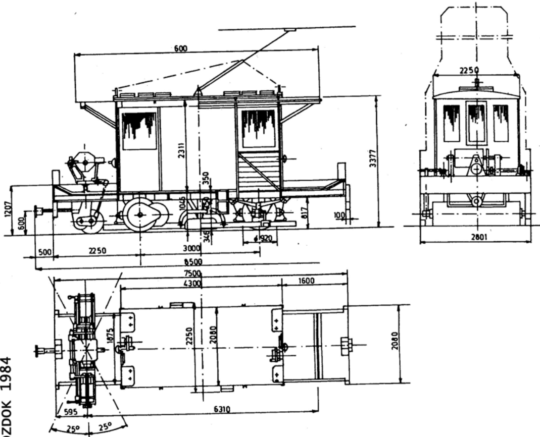
15.3. ábra Kardánhajtású villamosvasúti hóseprőmozdony jellegrajza
